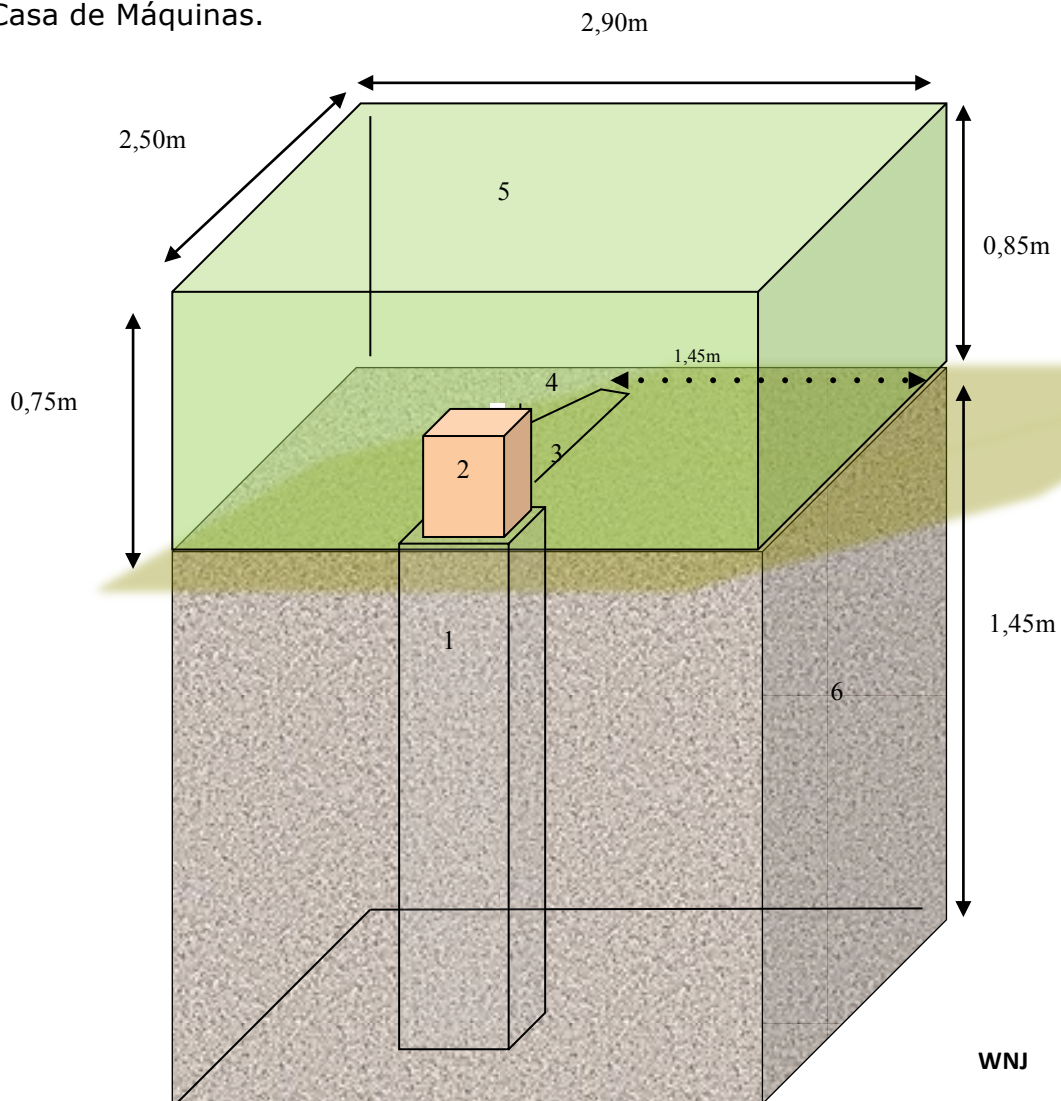
1 Bancada. 2 Máquina. 3 Braço. 4 ponta do braço. 5 Caixa. 6 Fosso.
